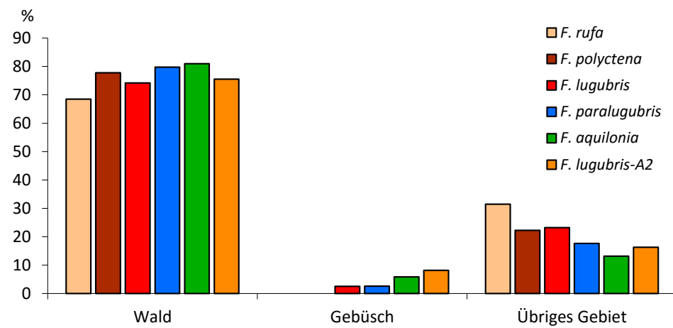
Abb. 4: Verteilung der Standorte der Nesthaufen der einzelnen Arten nach Vector25. Anzahl Beobachtungen: F. rufa : N=73, F. polycтена : N=35, F. lugubris : N=411, F. paralugubris : N=315, F. aquilonia : N=273, F. lugubris-A2 : N=49.
